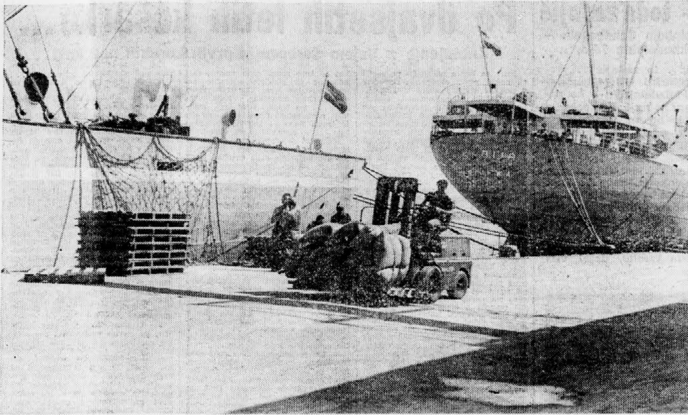
MEHANIZACIJA V LUKI KOPER — Ker je koprška luka urejena predvsem za promet z generalnim tovorom, ki zahteva vestno manipulacijo, skrbi predvsem za transportno mehanizacijo. Tako ima 24 mehaničnih transportnih trakov, 27 viljarjev in 10 traktorjev s 40 traktorskimimi priklopniki, za pretovor žita pa ima pnevmatično razkladalno in transportno napravo. V zaprtih skladiščih je zdaj 32.500 m 3 skladiščnega prostora.
