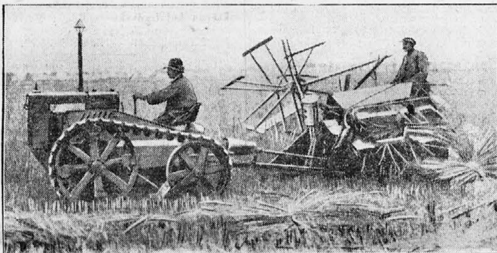
Stroj, ki žanje in veže snope
