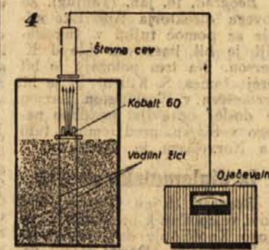
Shema merilca višine tekočine v zaprtih tankih.
