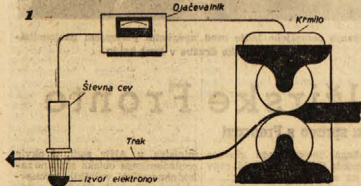
Shema merilca, ki preko ojačevalnika sam krmili razdaljo valjev. Trak ima tako ves čas enakomerno debelino.
