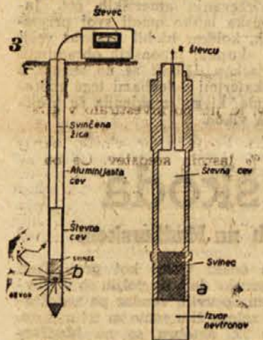
Sonda za meritve množine nafte ali vode v zemlji. Meritev vlage v zemlji: Aluminijasta cev, v kateri je sonda, zabijemo v zemljo. Izvor v sondi oddaja hitre nevtrone, ki letijo v zemljo. Zaradi trka z vodikovimi jedri opišejo nevtroni cikcakasto pot, izgubijo energijo in kot počasni nevtroni priletijo na števec. Na sliki je vršena pot enega samega nevtrona.
