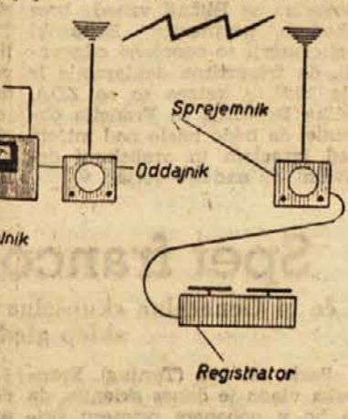
Shema naprave, s katero merimo na daljavo množino vode v snegu
