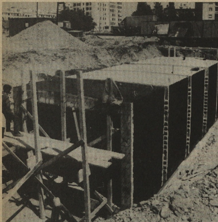
Škatlasti betonski elementi podhoda za pešce pred montažo.
