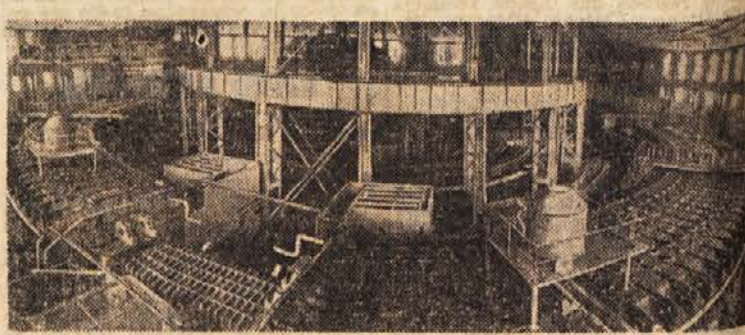
Pogled v elektrofizikalni laboratorij Akademije znanosti ZSSR. Na sliki vidimo sinhrotron za 10 milijard elektronvoltov
