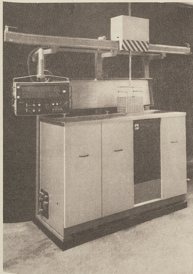
Iz Tozda Strojegradije — Programirana naprava za ultrazvočno čiščenje kovinskih delov, ki jo izdelujejo v kooperaciji z Inštitutom za elektronsko in vakumsko tehniko iz Ljubljane.
