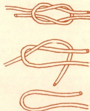
Križni vozel
