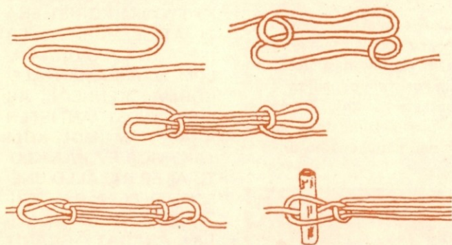
Skrajševalni vozli
