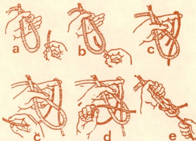
Tkalski vozel
