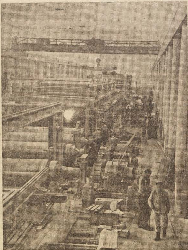
Pogled v strojno dvorano tovarne rotacijskega časopisnega papirja v Vidmu, kjer se že vidi obrisi velikega papirnega stroja, dolgega 110 m.
