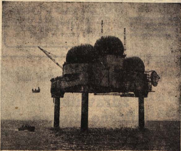
Okoli 120 km severovzhodno od ameriške atlantske obale je »radarski otok«, na katerem ima ameriško vojsko letalstvo opazovalnico. Ogrodje umetnega otoka ima obliko trikotnika s 60 m dolgimi stranicami
