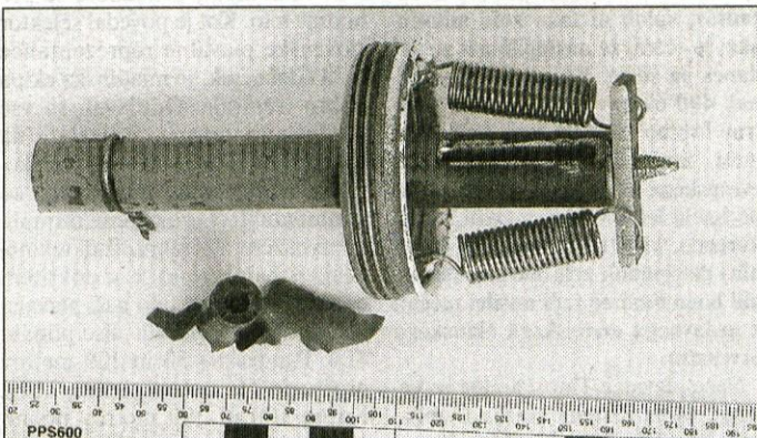
Doma izdelan detonator.
