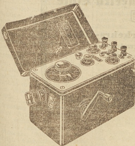
Neuzeitliches Betriebs-Meßgerät im Blechgehäuse: Erdungsmesser zum Nachprüfen der Erdung von Hochspannungsmasten usw.
