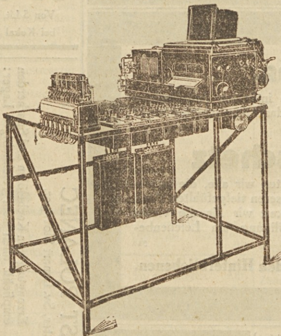
Eine Spitzenleistung der Meßtechnik: Siemens-Universal-Oszillograph zum Aufzeichnen schnell veränderlicher elektrischer und mechanischer Vorgänge.
