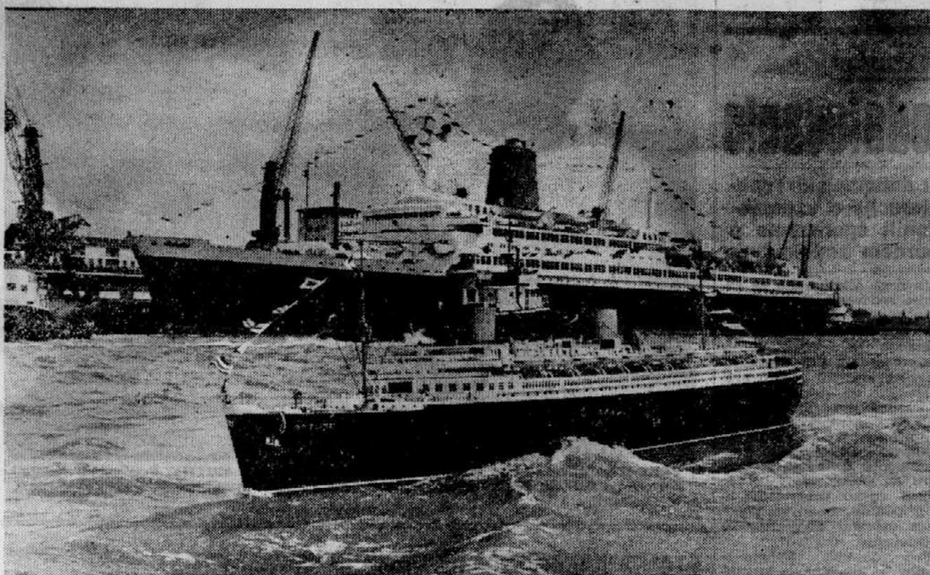
Dobrih dvajset metrov dolgi osemtonski model stare žezoceanske potniške ladje »Bremena« je pred dnevi ob izlizu Wesere nekaj časa spremljal svojo novo »mamno« istega imena, ki se loči od stare (model v ospredju) tudi po dveh dimnikih. Po zaslugi motorjev, ki imata vsak po 38 KM, zmora barčica do 14 vozlov na uro. Foto AP
