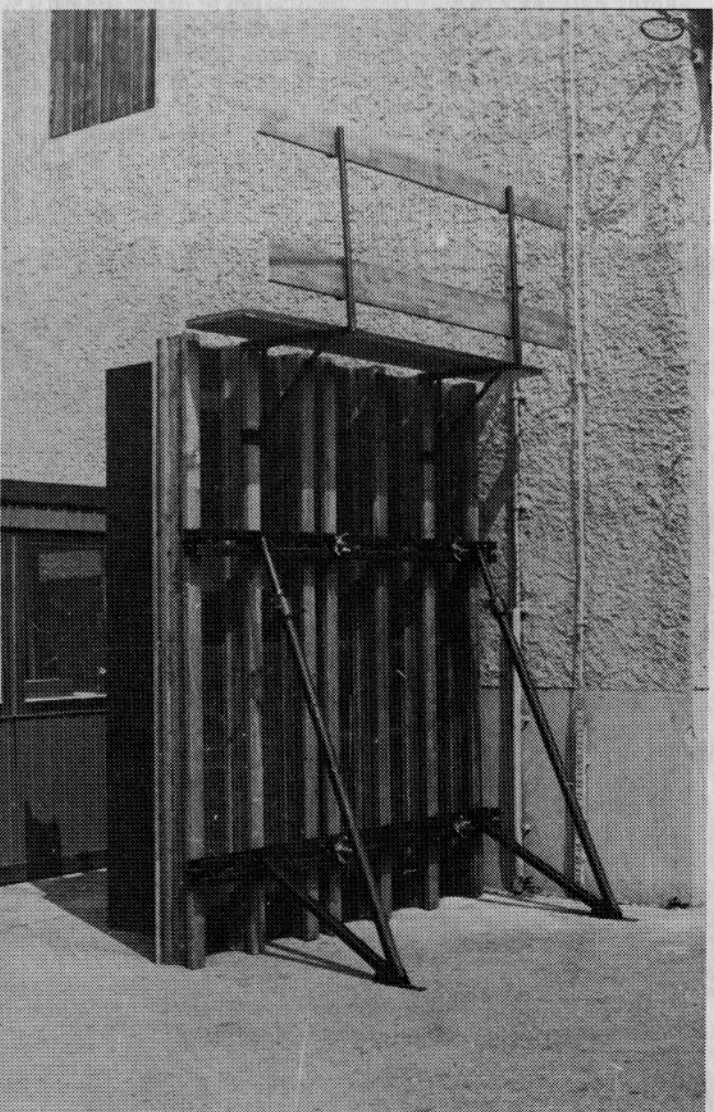
Primer sestave opaža za steno
