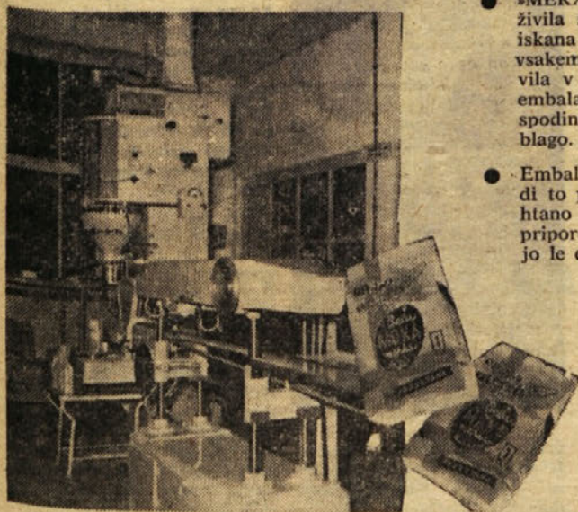
Posnetek iz celjskega trgovskega podjetja »MERX«: embalirni stroj »Hesser« za embaliranje moke in mletvskih izdelkov
