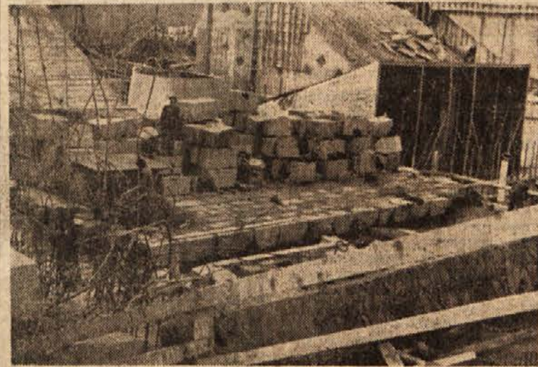
Z velikimi betonskimi kockami oblagajo pretočno polje
