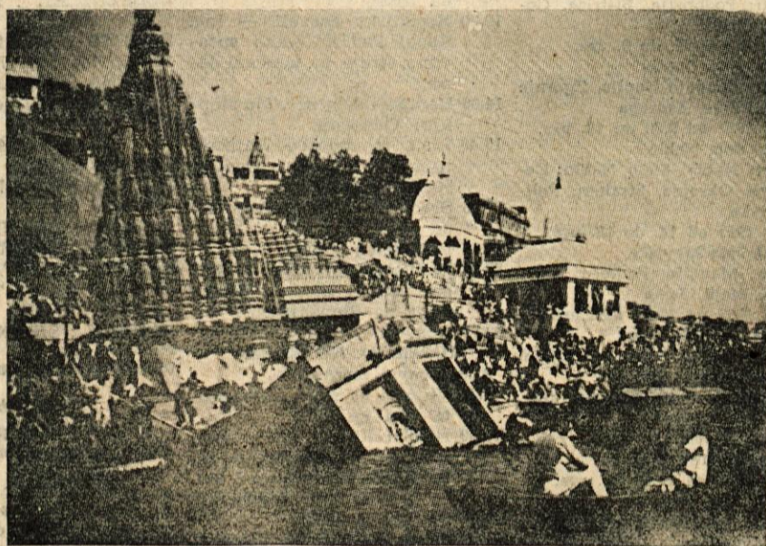
V monsumskem deževju Ganges preplavi pogrezojoče bregove
