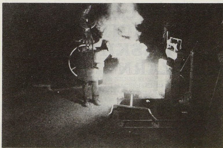
Tehtanje taline in dodajanje magnezija v livarno I
