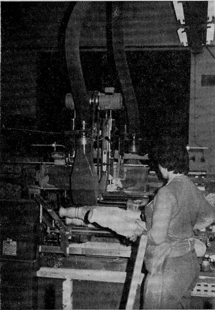
Brusilni stroj za brušenje struženih elementov. Na njem delavka brusi noge pogradov. Ko so obdelovanci strojno obrušeni, jih je treba na drugem stroju še ročno obrusiti
