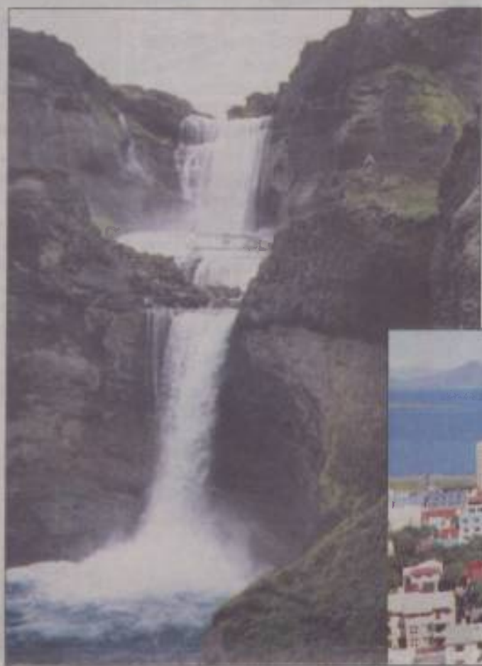
Slap Ofaerufoss, eden mnogih na Islandiji. Pred leti ga je še dodatno krasil most, ki pa ga je zima podrla.
