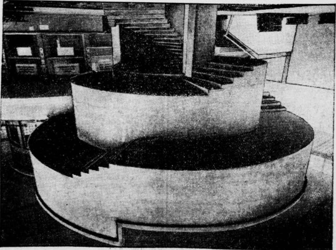
Spiralno stopnišče iz železobetona, vltito v en gam kos.
