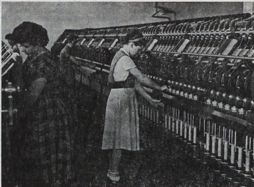
Gill stroj za predenje konoplje
