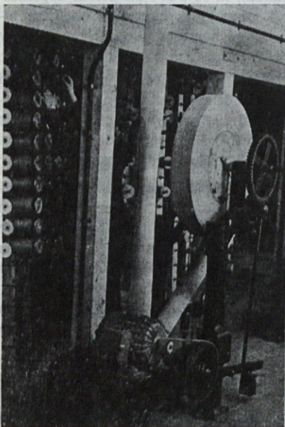
Detajl s stroja za okroglo tkanje gasilskih cevi
