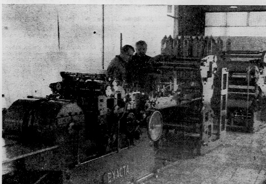
Stroj za pakiranje vrečk, izdelek tovarne »Gartemann & Hollmann« iz Bielefelda, med montiranjem na Gospodarskem razstavišču. Stroj bo med razstavo ves čas v pogonu, tako da si bodo obiskovalci razstave lahko ogledali mehanizirano pakiranje.
