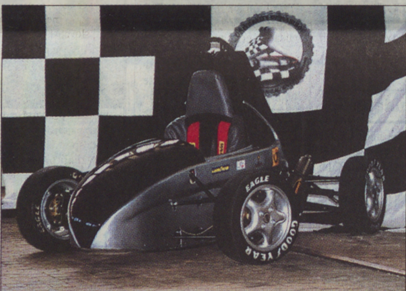
Na Fakulteti za strojništvo so izdelali tudi formulo, ki ima 600 m 3 dirkalni Hondin motor s turbinskim polnjenjem. Pospešek dirkalnika od 0 do 100 km/h je 4,8 sekunde, doseže pa hitrost 200 km/h.
