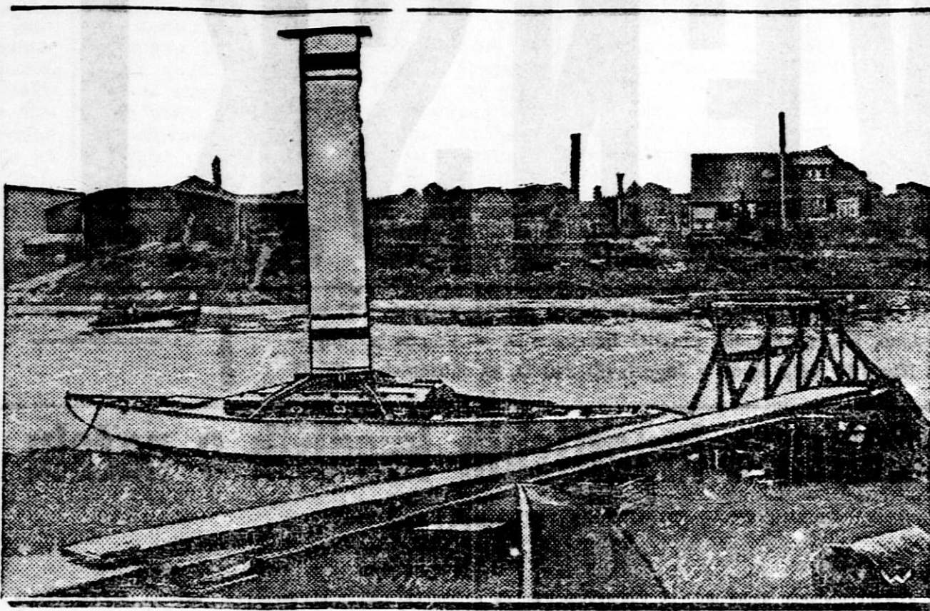
PRVA FLETTNERIEVA ROTTOR-JADRNIC, ki jo je zgradila tvrdka Burmester v Bremenu, je dosegla pri poskuhi vožnji prav lepe uspehe.
