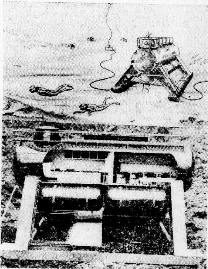
PODVOJNI LABORATORIJ — Prihodnje leto maja nameravajo pri skalnatem otoku Helgoland spustiti v morje podvodni laboratorij, v katerem bodo štirje znanstveniki raziskovali morsko dno v globinah 20—45 m pod gladino. Med drugim bodo skušali ugotoviti, kako reagirata srce in ožilje na telesni napor v celici pod pritiskom in izven nje ter na daljše bivanje v mrzli vodi. Podvodna hiša ima prostornino 46 kubičnih metrov. Slika kaže model in risbo podvodnega laboratorija s telefonsko in televizijsko zvezo z obalo.
