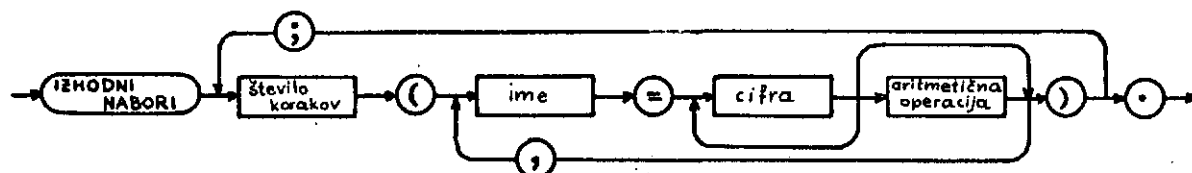
Slika 15. Stavak IZHODNI NABORI
