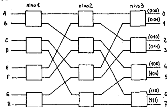
Slika 3.2.2.3. Delta mreža 8x8.
