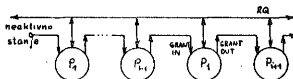
Slika 3.2.1.a. Serijska metoda.
