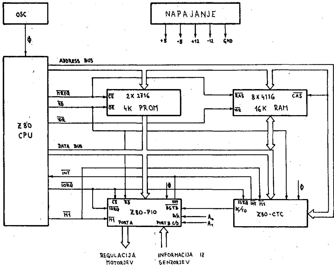
Slika 4: Bločni diagram mikroračunalniškega kontrolnega sistema
