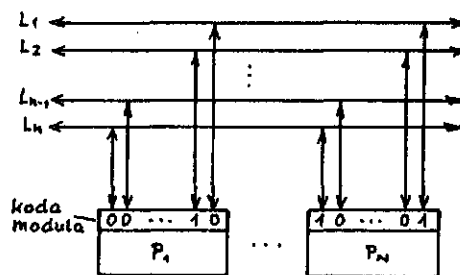
Slika 3.2.1.c. Samoizbirni mehanizem.
