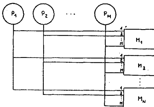
Slika 3.2.3.1. Sistem s pomnilniki z več vrati.
