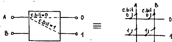
Slika 3.2.2.2. "Crossbar" vezje 2x2.
