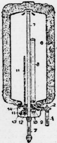
Pokročni presek boilerja:
