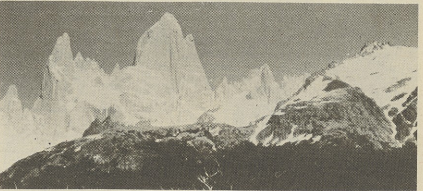
Pogled na mogočno jugovzhodno steno patagonskega očaka Fitz Roya
