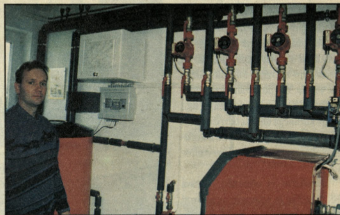
Radovan Novak ob svoji krmilni napravi KRN 3000 v kotlovnici
