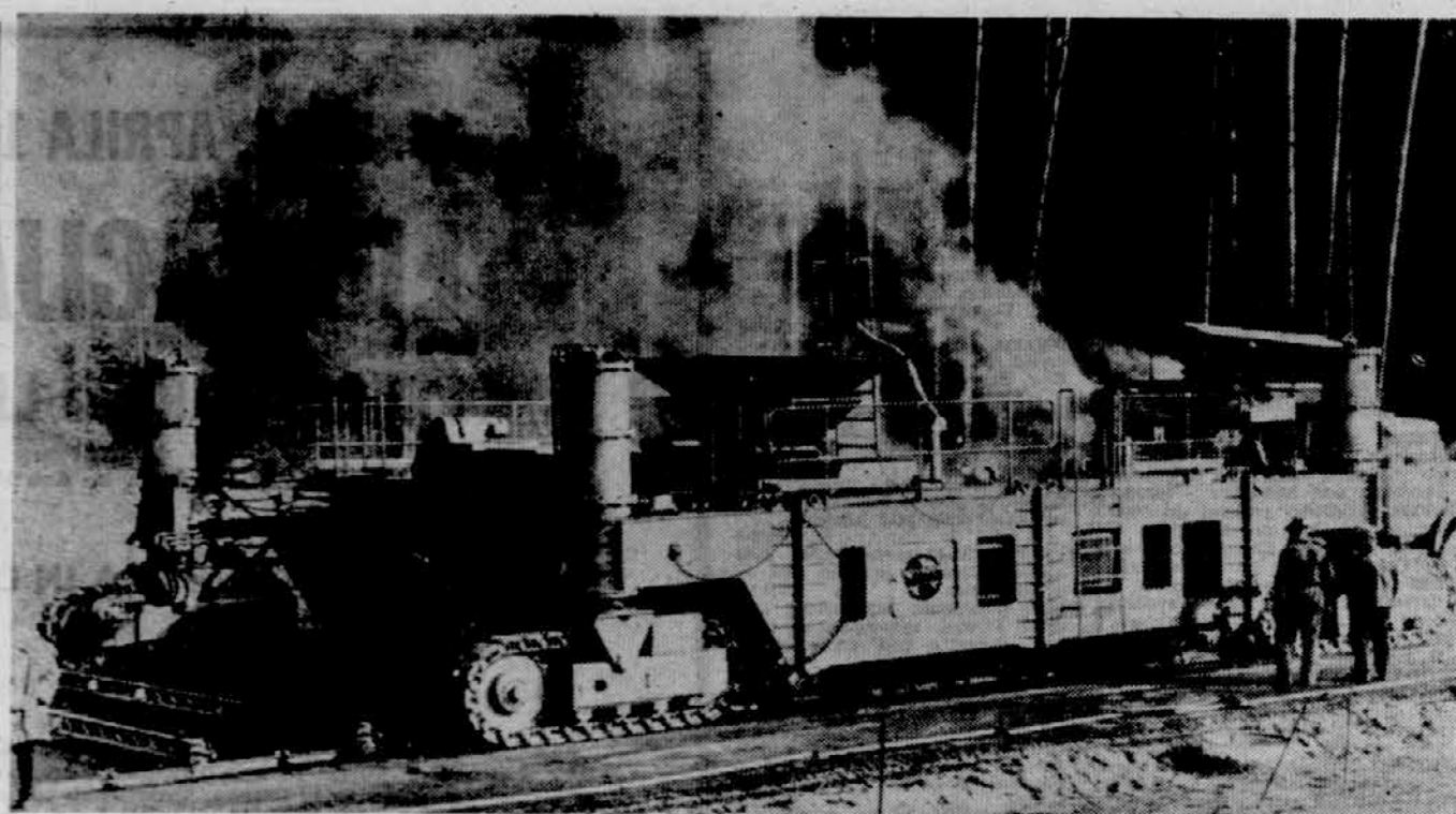
ASFALTNI TRAK SE NAGLO DALJŠA — Lani so zgradili v ZRN skoraj 300 kilometrov novih avtomobilskih cest, za letos jih napovedujejo še več po zaslugi novih gradbenih strojev. Velik stroj na sliki asfaltira v desetih urah 15,23 metra širok cestni odsek v dolžini 3,5 kilometra.
