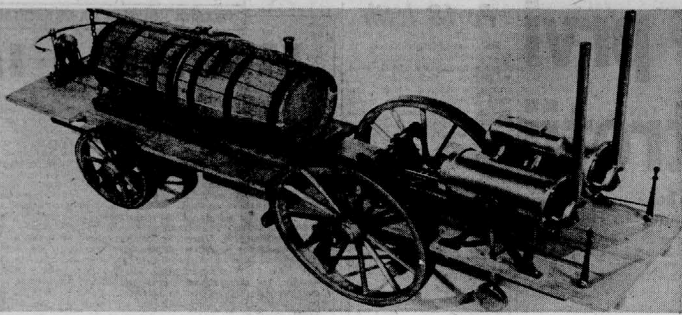
RESSLOV PARNI AVTOMOBIL — ALI CESTNA LOKOMOTIVA, KAKOR HOCETE... Fotoarhiv Dunajskega tehniškega muzeja
