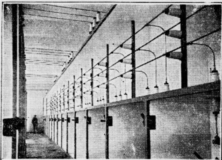
Zgradnja 20.000 voltov v transformatorski postaji v Črnučah, odkoder se cepijo daljnovodi v posamezne kraje
