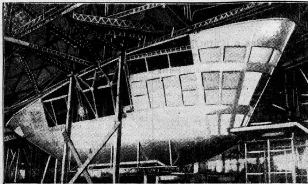
Amerikanci grade ogromen zrakoplov sistema »Zeppelin«
