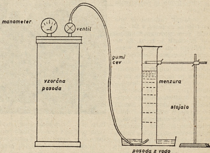
Sl. 1 NAPRAVA ZA MERJENJE PLINA V PREMUGU
