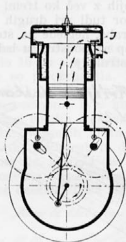
Slika 8 Izpušni takt.
