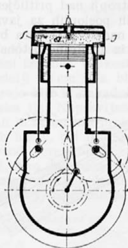
Slika 7 Delovni (eksplozijski) takt.
