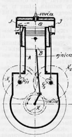
Slika 5 Izvalni takt.
