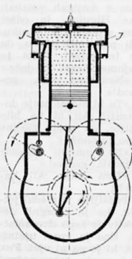
Slika 6 Kompresijski takt.
