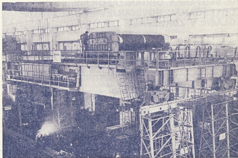
Dvigalo 180 Mp za HE Hemren Dam v poizkusni montaži (Foto: J. Ziebnik)
