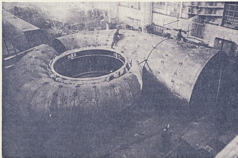
Druga špirala za HE Hemren Dam (Foto: J. Ziebnik)
