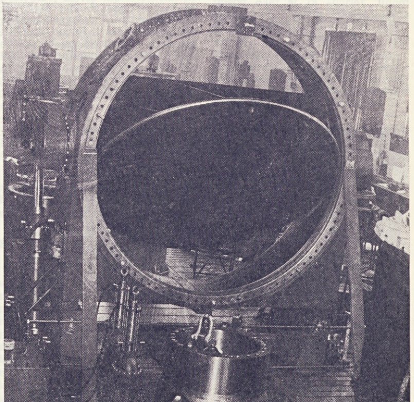
Predturbinska loputa premera 5000/4800 mm za HE Hemren Dam v Iraku (Foto: J. Jereb)
