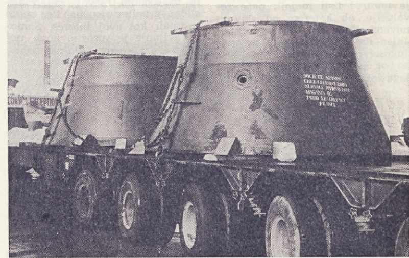
HE Čakovec — konusa turbine na začetku poti (Foto: J. Žlebnik)
