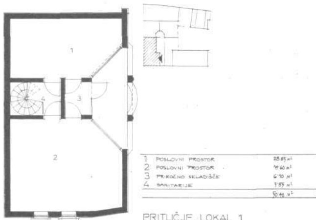
PRITLIČJE, LOKAL 1
