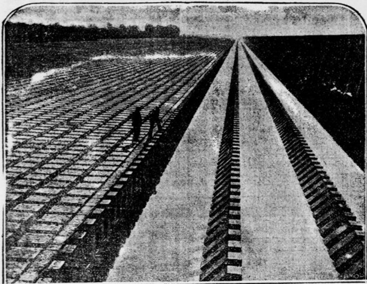
Z velikanskimi nasipi in pragovi iz profiliranega železobetona, ob katerih naj bi se zlomila moč deroče reke so zavarovani bregovi Mississippija, vendar tudi ti ne morejo zmerom zdržati vodnega pritiska
