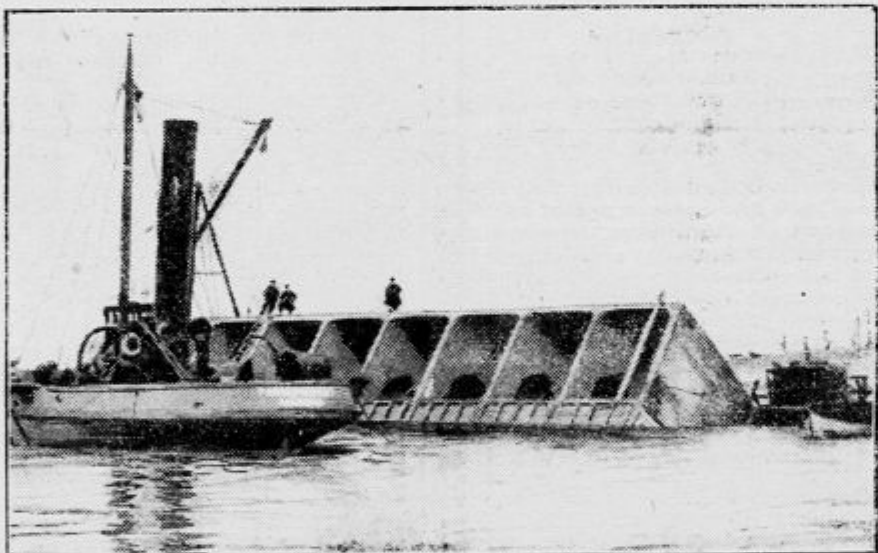
Plavajoča železobetonska skrinja pred pogreznjenjem v morje.
