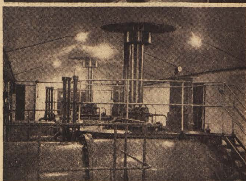
Strojnica v prerezu (od zgoraj navzdol): razvodne naprave nad podzemno strojnico — druga slika predstavlja strojnico s prvima dvema generatorjema, po 7500 kVA — tretje nadstropje pod zemljo: hidromehanske naprave, ki avtomatično, lahko pa tudi ročno regulirajo dotok vode na turbine in vse ostalo. — Najnižje so montirane Francis spiralne turbine z navpično osjo. Vse razen generatorja je izdelal »Litostroje«.
