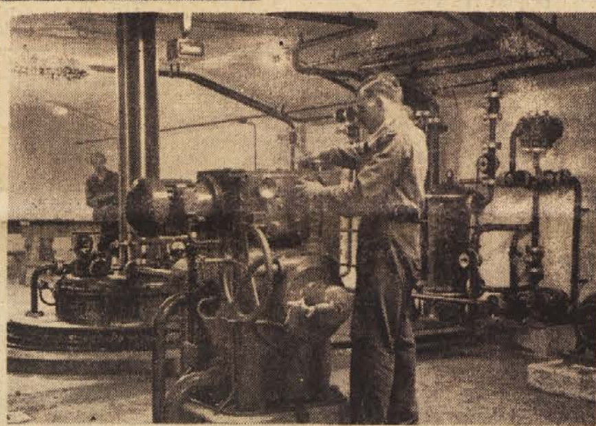
Servomotor za odpiranje oziroma zapiranje dovodnih lopatic
