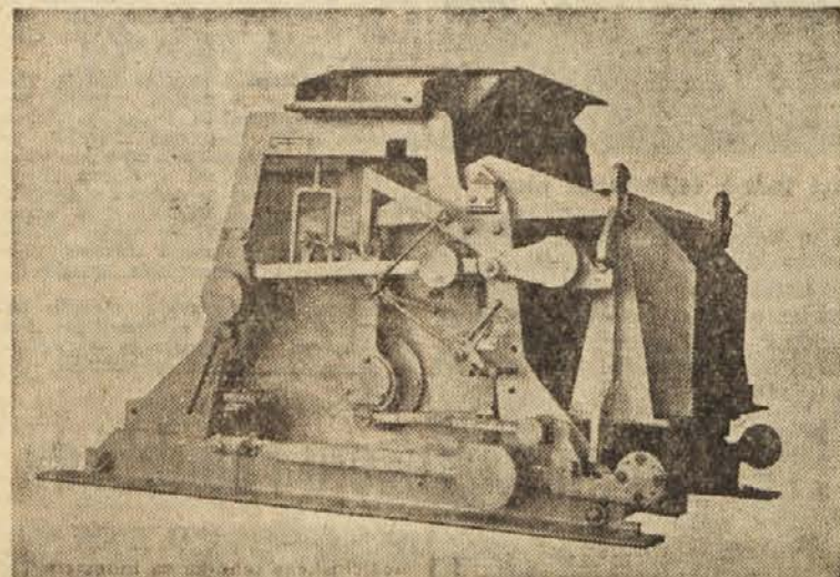
Tehnica na transportnem traku za potrebe rudarstva in tovarna cementa. Prototip je izdelal leta 1954 Veselak Avgust. Sedaj novi serijski proizvod
