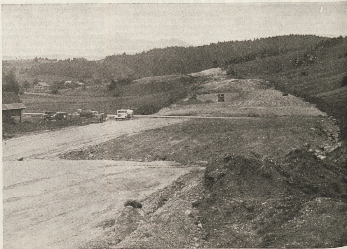
Težki gradbeni stroji so že močno spremenili izgled zemljišča pri UNCU, kjer bo tekla nova avtomobilska cesta. Dela lepo napredujejo. Specializirano gradbeno podjetje Mavrovo iz Skopja gradi odsek 12 km dolge trase, katere del vidite na fotografiji. Več o cesti, tem podjetju in drugih zanimivostih iz te velike gradnje pa bomo objavili v prihodnji številki obzornika
