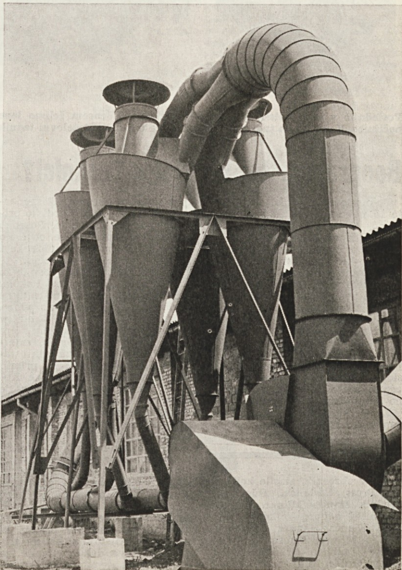
Nove ekshavstorske naprave s cikloni v Tovarni lesnih izdelkov Stari trg
