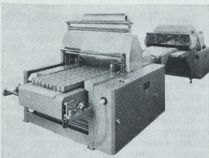
Beckov pakirni stroj s komoro za skrčenje folije
