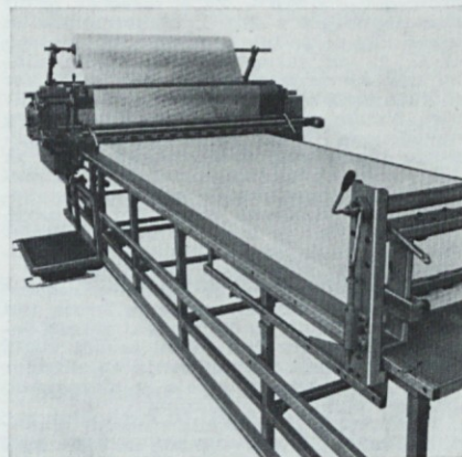
Avtomatsko pokladanje plasti blaga
