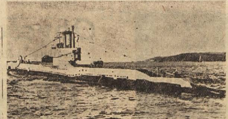
Na sliki vidite angleško podmornico, ki se je pred dnevi potopila v pristanišču Harbour. Vzrok nesreče je bila eksplozija, ki je nastala na napravah za istrežitev torpedov. Življenje je izgubilo 13 mornarjev. Podmornica leži 10 metrov globoko. Te dni jo bodo dvignili z morskega dna. Nato bodo še točneje ugotovili vzrok nesreče
