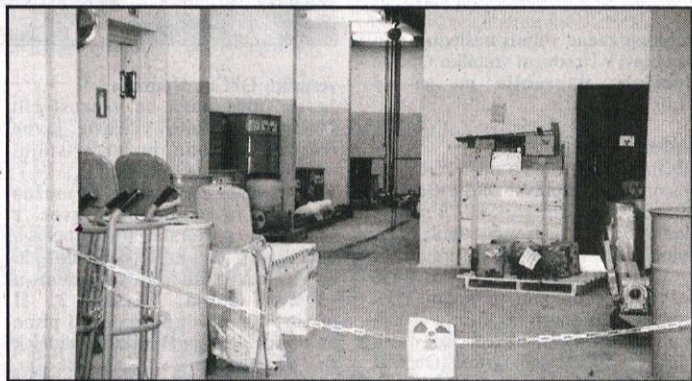
Pogled v skladišče radioaktivnih odpadkov
