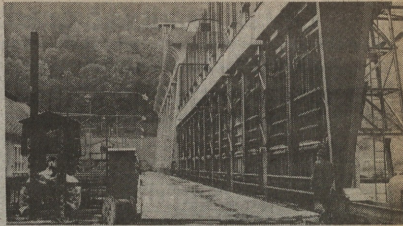
Generatorji HE Fala so dajali elektriko šest desetletij, tako da gredo v zaslužen pokoj. Jez in zapornice pa bodo po prenovi služili novi strojnici.
