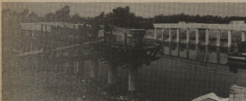
Na mostu čez Ljubljano se odstranjujejo opaži za desni opornik, tako da se bo tudi na tem objektu kmalu začela montaža nosilcev.
