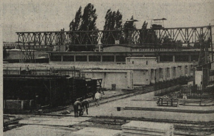
Nosilci so pripravljeni za prevoz do deponije ob železnici, nato pa v Višegrad in Ljubljano
