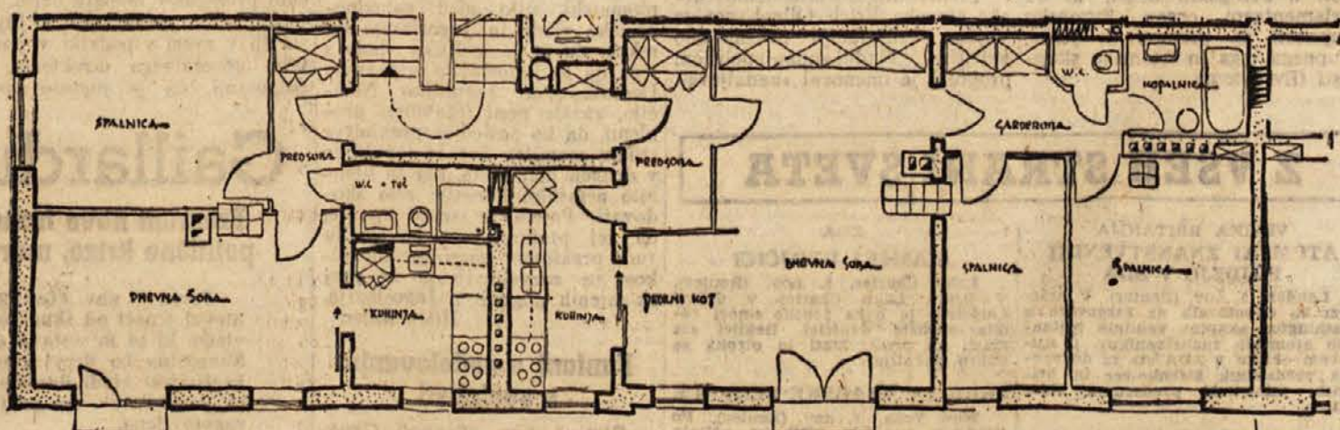
Načrt ing. arh. Iva Štruklja, po katerem grade v Savski koloniji štiri stanovanjske bloke z eno- in dvosobnimi stanovanji
