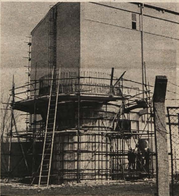
Nova tovarna magnefitne celuloze v Krškem bo dokončana do jeseni. Zima ne ovira gradbenih del. (Foto: Jožica Teppey)
