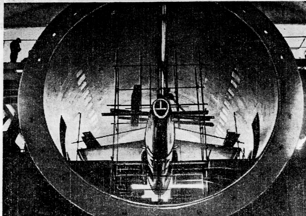
Pogled na največji vetrovni kanal na svetu pri mestu Modane pod Mount Cenisem ob francosko-italijanski meji. Model letala, ki ga aerodinamične lastnosti žele preizkušati v tem viharniku, pritrjuje na 328 ton težak premični podstavek.
