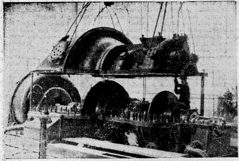
Velika parna turbina termoelektrarne v Trbovljah med obnovitvenimi deli
