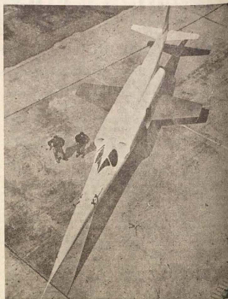
Ameriško vojno letalstvo je nedavno prvokrat objavilo sliko novega dvomotornega reaktivnega letalca X-3. To letalo bo letalo na dolgih progah. Preizkušali so ga leto dni v preizkuševalnici letalske baze v Kaliforniji in poskusni poleti so pokazali vse njegove vrline. Letalo je dolgo 18,9 m in podobno meču. Samo instrumenti za preizkušanje tehtajo 600 kg, razen tega pa ima še več standardnih instrumentov modernega reaktivnega letalca. Doseže pa hitrost 3200 km na uro.
